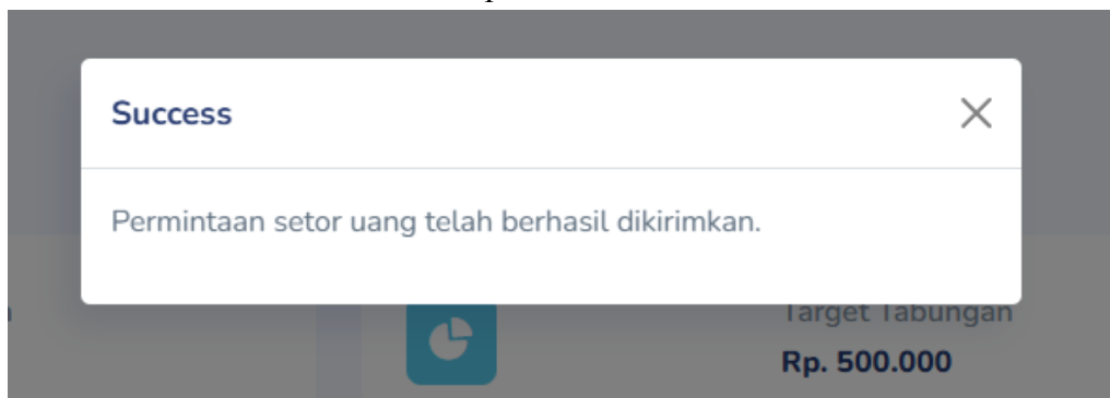
Gambar 3.6 Notifikasi Success
