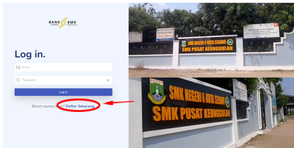
Gambar 1.2 Halaman Login
