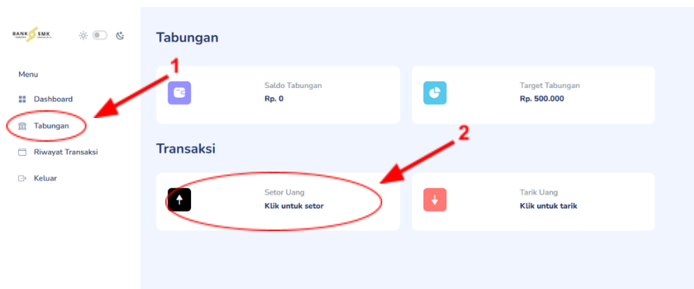
Gambar 3.4 Halaman Tabungan
