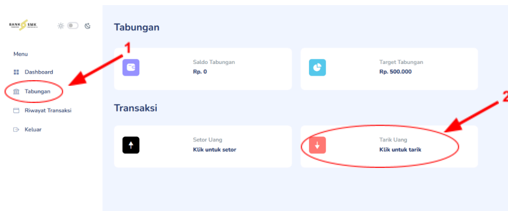
Gambar 4.4 Halaman Tabungan
