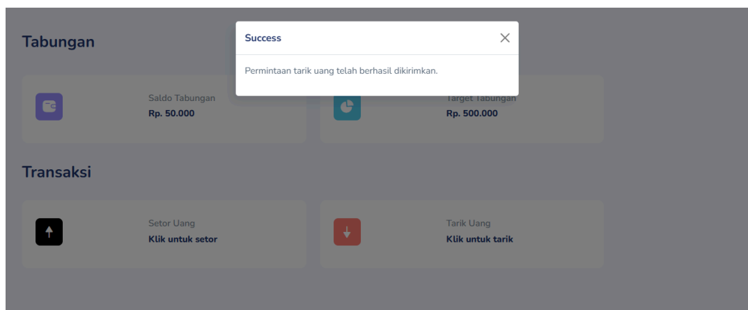
Gambar 4.6 Notifikasi Success
